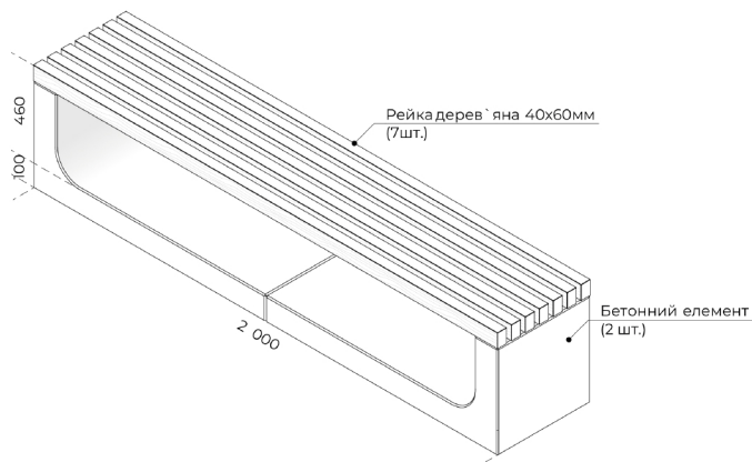
Схема лавки
