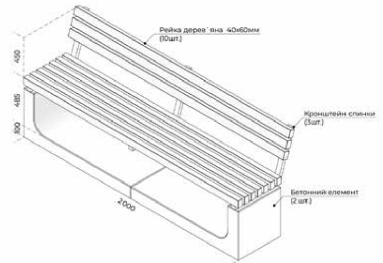
Схема лавки
