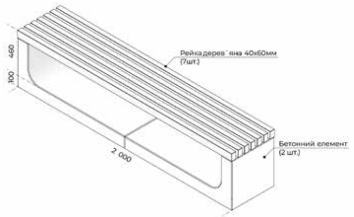
Схема лавки
