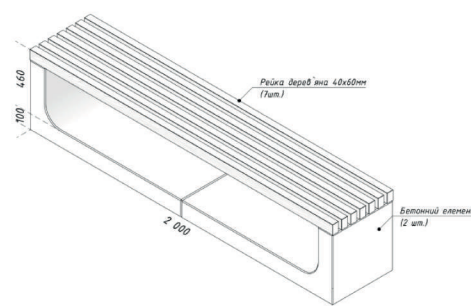
Схема лавки без спинки
