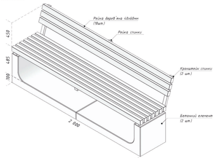
Схема лавки
